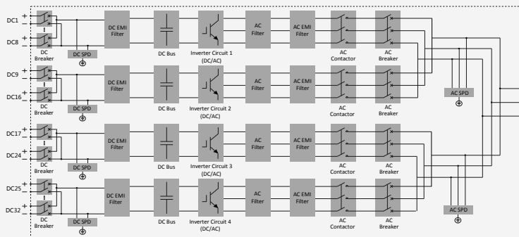
Circuit Diagram / 단선도
